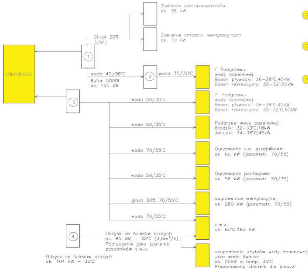
Zał. 1 SCHEMAT BLOKOWY ROZWIĄZAŃ PRZYGOTOWANIA CIEPŁA I CHŁODU DLA PROJEKTOWANEJ PŁYWAJNI
